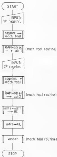
Afb. 5-1 Flowchart van het BASIC-programma 'blokdol'
